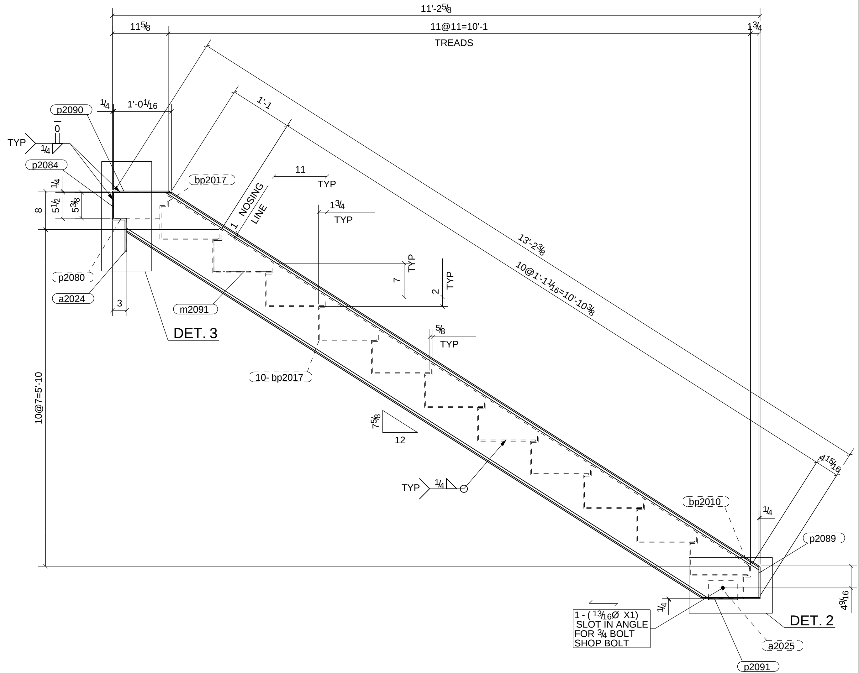
B - B
